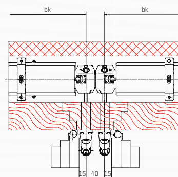
Actionnement à manivelle
